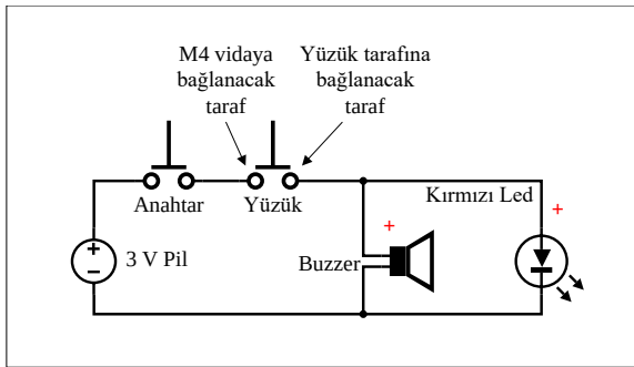
Şekil 6.6: Devrelerin Şeması
