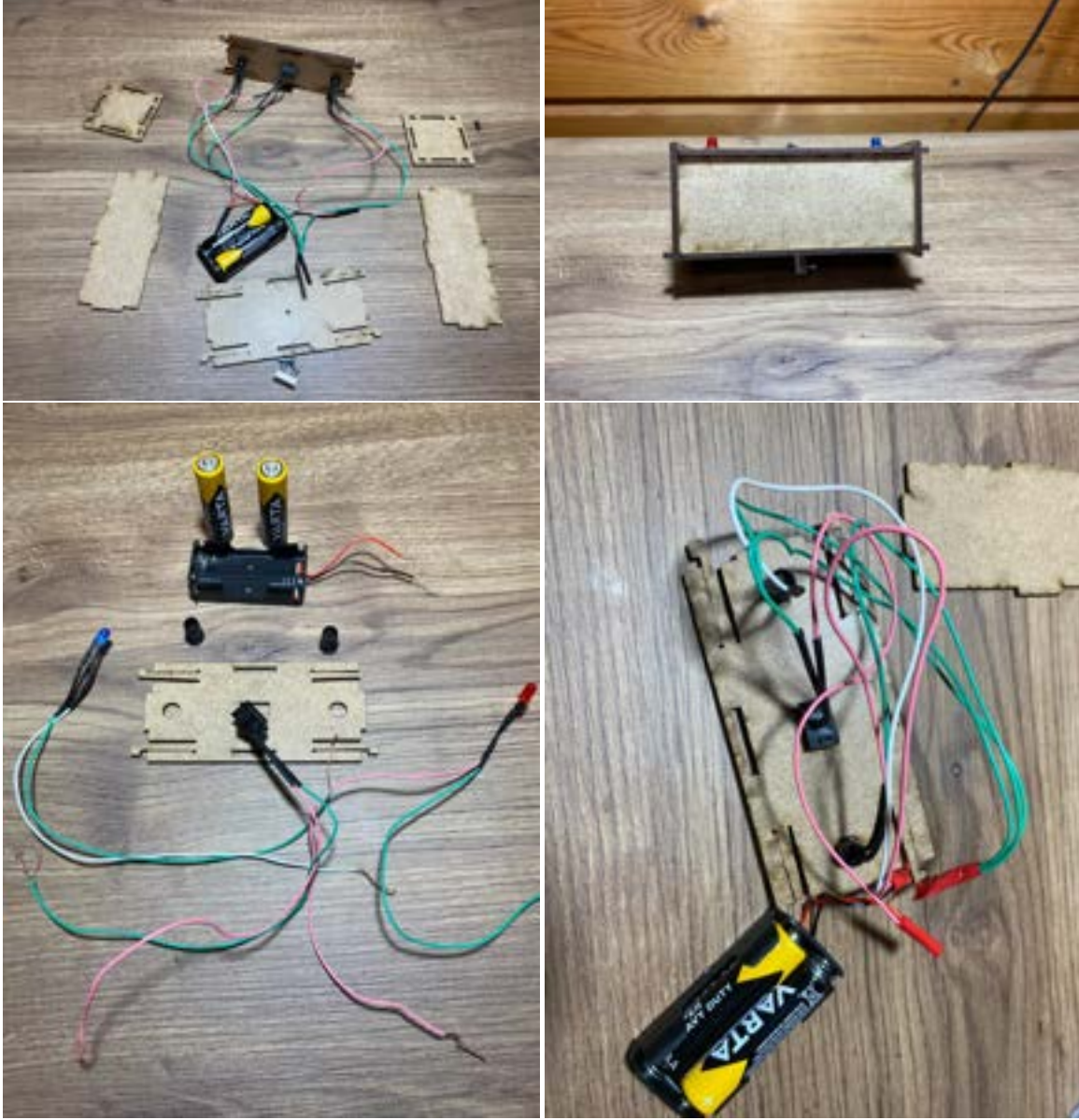
Şekil 6.5: Led ve yuvasının montajı
