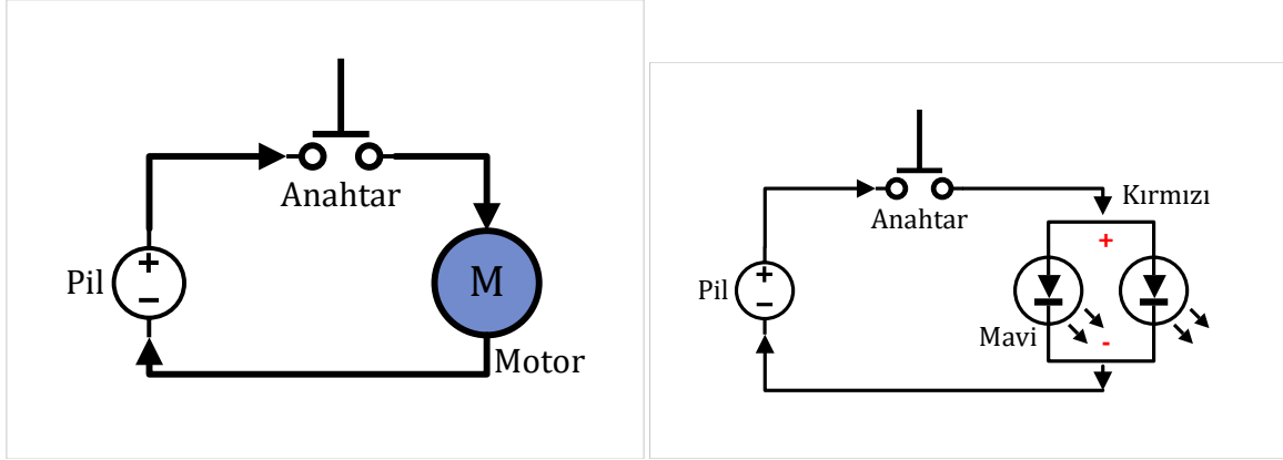
Şekil 6.7: Devrelerin Şeması
