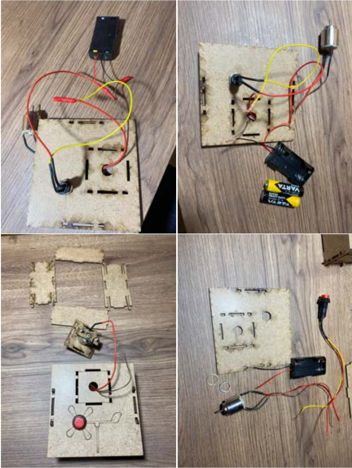
Şekil 6.4: DC Motor bloğunun montajı
